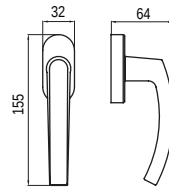
YFZ06 Inward-open spindle handle
