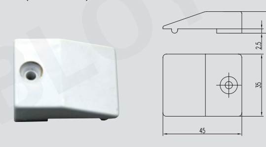
LB13 (Sash Lifter)
