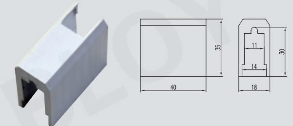
BB 88 (Bumper Block)
